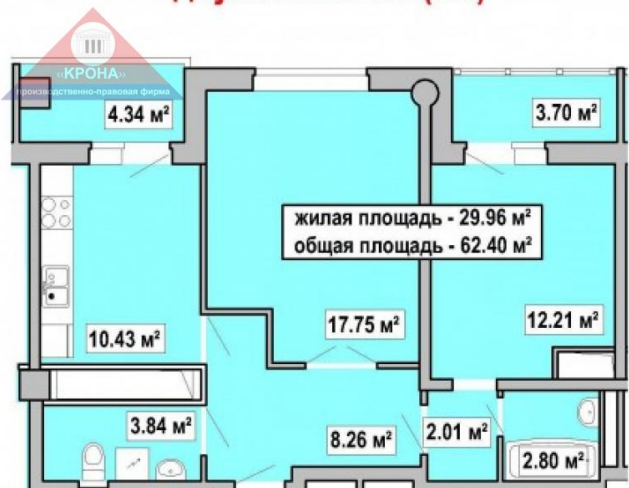
двухкомнатная (II-5)
